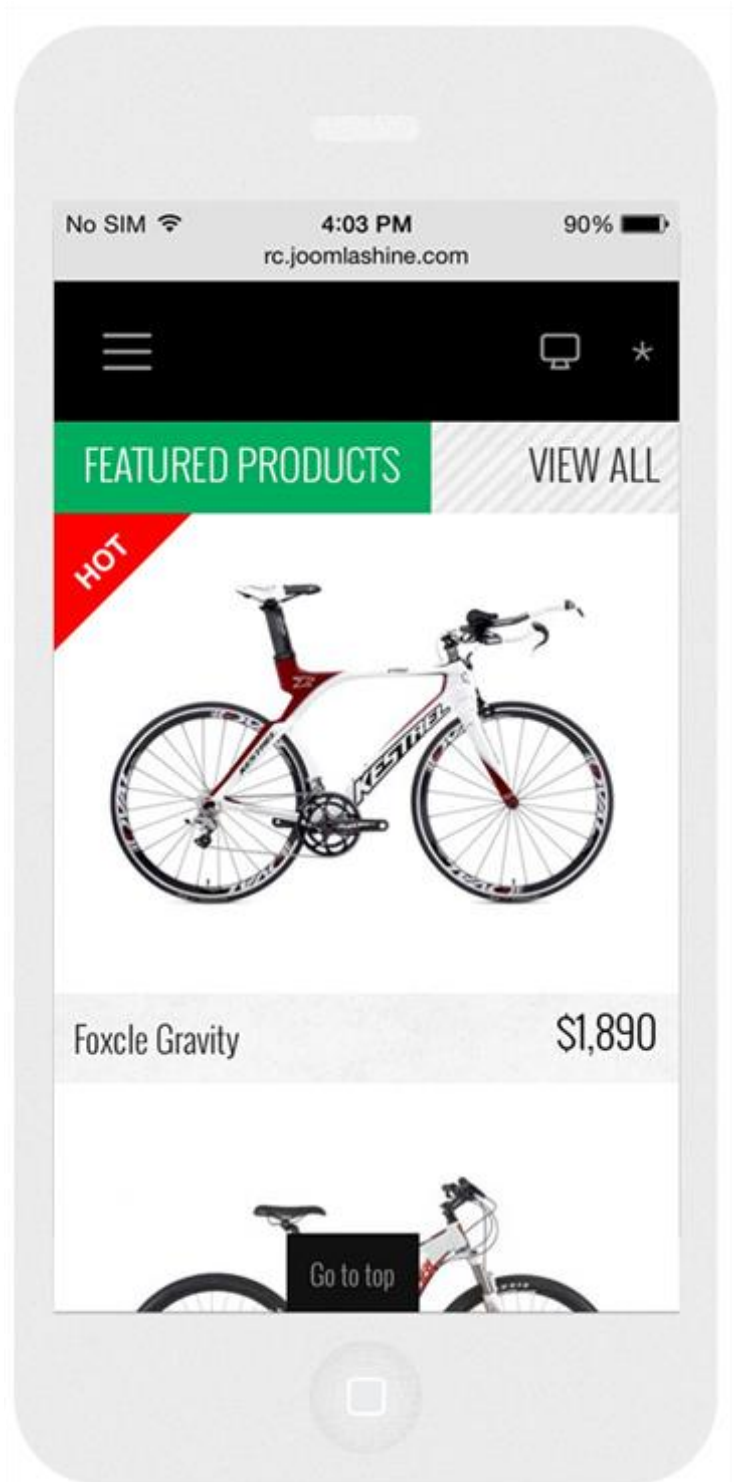
1-column module
